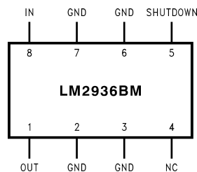
Figure 5. 8-Pin SOIC (D) Top View
